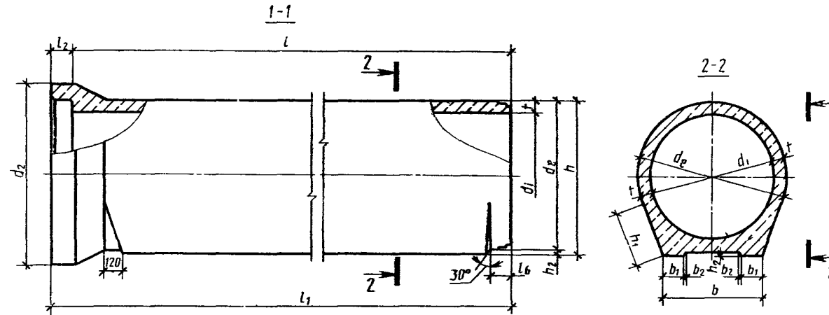
Продольный разрез стенки трубы
