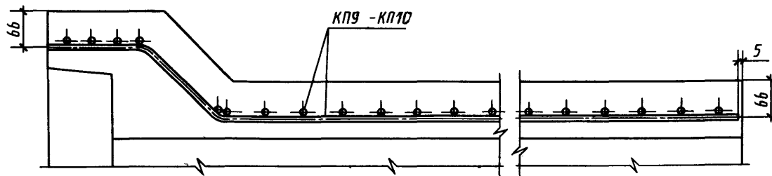
Деталь армирования стенки трубы
